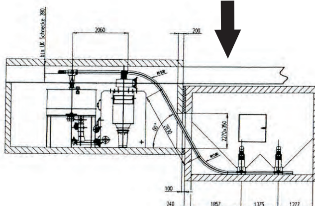
von Nolting erstelltes Pelletlager (Unterboden)
